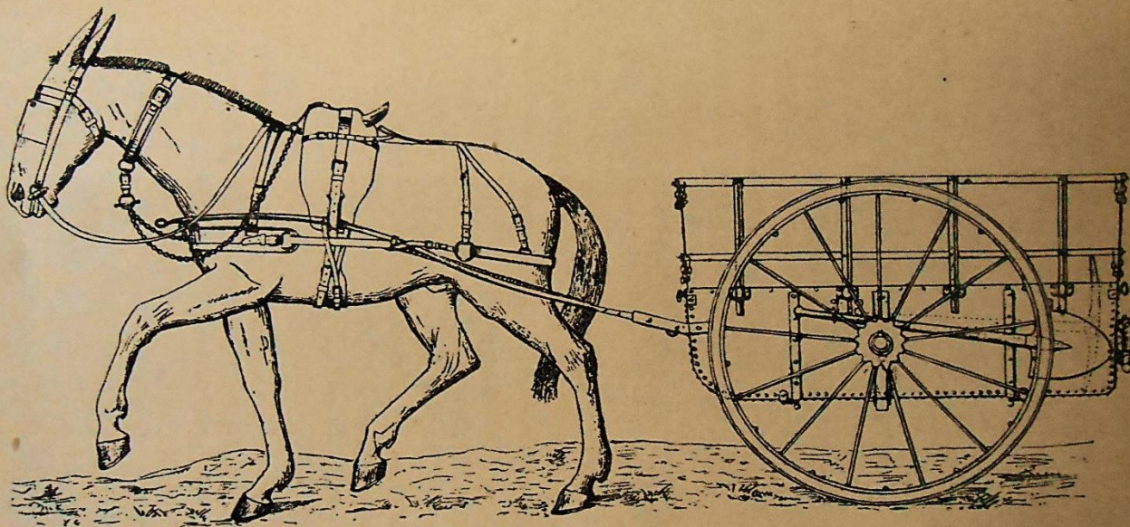
La voiture Lefebvre en tôle d'acier pèse, avec les ridelles et les brancards, 142 k , et a 1 m ,04 de voie; un mulet traîne avec elle une charge réelle de 300 à 400 k . Un deuxième modèle à voie étroite (0 m ,70) est en essai; la voiture étant plus longue, la capacité est la même. Enfin une troisième voiture est actuellement en essai au Dahomey; cette dernière en aluminium ne pèse que 61 k , a 0 m ,70 de voie et peut porter de 400 à 800 k . Les caisses enlevées des roues peuvent servir de bateaux plats pour l'établissement d'un pont de bateaux.
